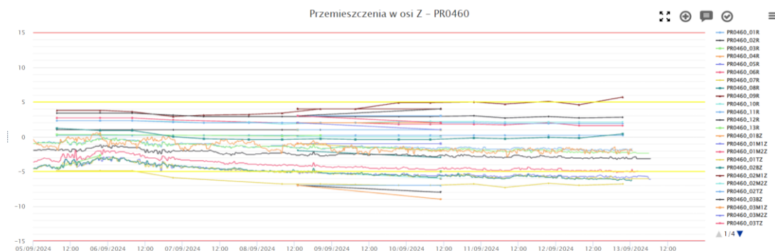
Rysunek 6-5 Osada budynku PR0460 – Geoscope
